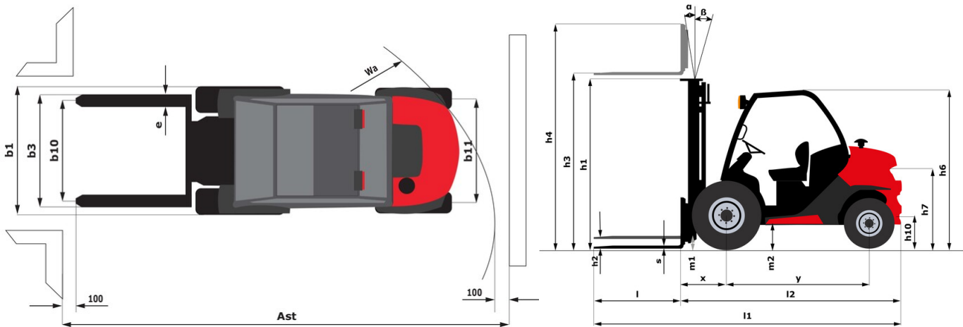
MC 18-4 ST5 - Schémas d'encombrement
