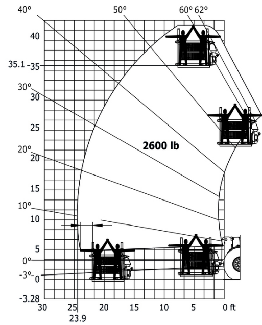
Machine sur pneus avec panier mine (Impérial)
