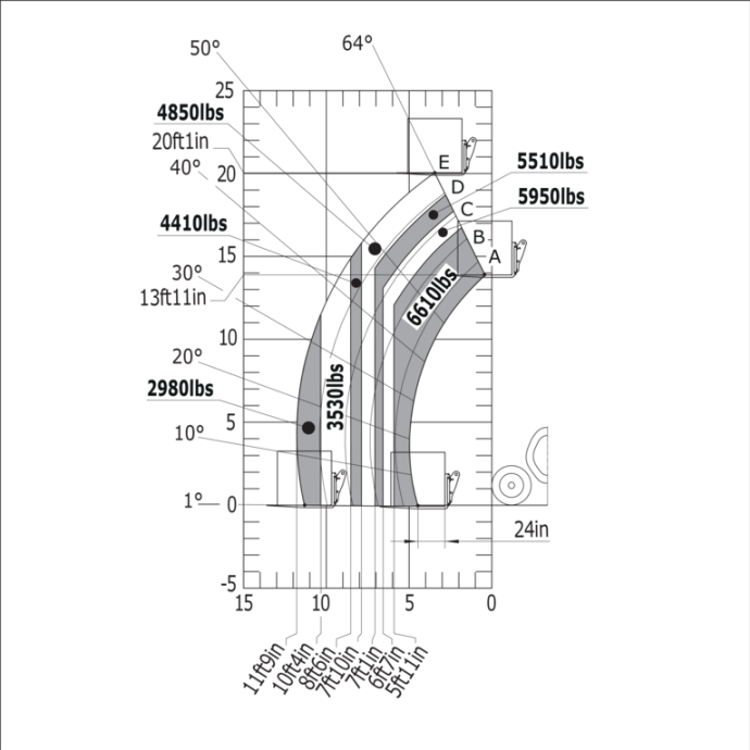
Machine sur pneus avec fourches CDG 600 mm (Impérial)
