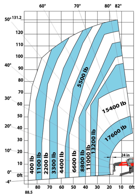
Machine sur stabilisateurs abaissés avec fourches Impérial
