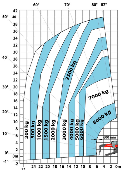
Machine sur stabilisateurs abaissés avec fourches
